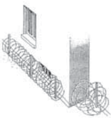
Figuur 201a: Draadversperring in dode hoeken
