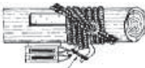
Figuur: Haakzekering
