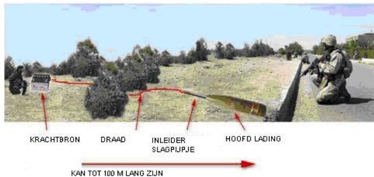
Voorbeeld Command wired IED (CWIED)
